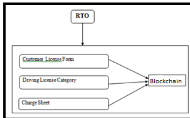
Fig. 3. RTO Module
