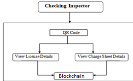
Fig.4.Checking Inspector Module
