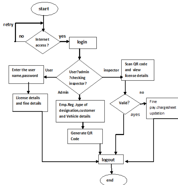
Fig. 2.Admin Module
