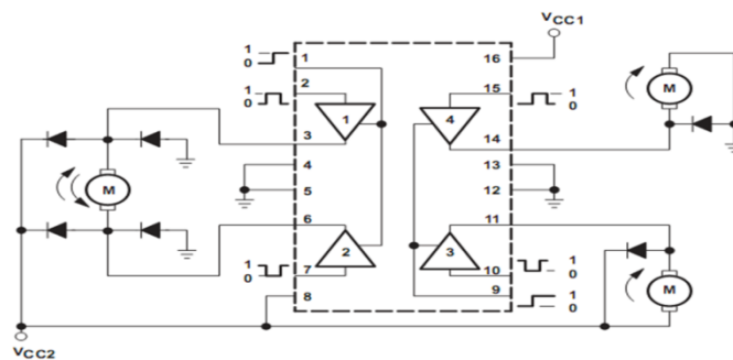
Fig. 6 L293D
