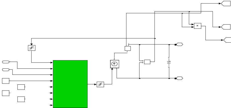
Fig. 5 Simulink Model For PV Module - I
