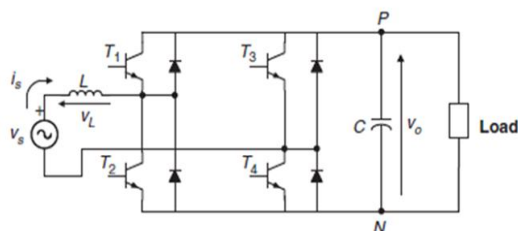
Fig. 1 Single phase Boost rectifier
