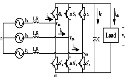
Fig.17.Three Phase PWM Rectifier
